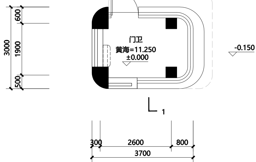
2#楼 一层平面图
