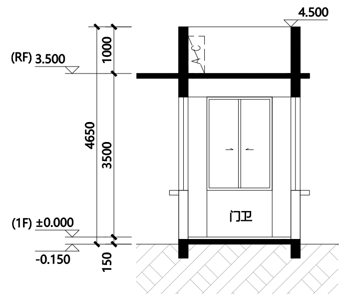
2#楼 1-1剖面图
