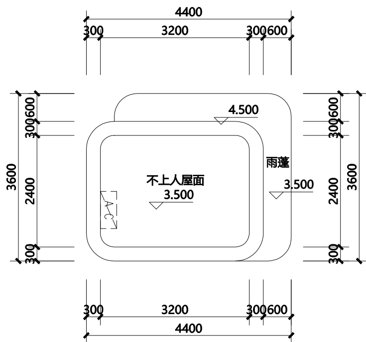
2#楼 屋面层平面图
